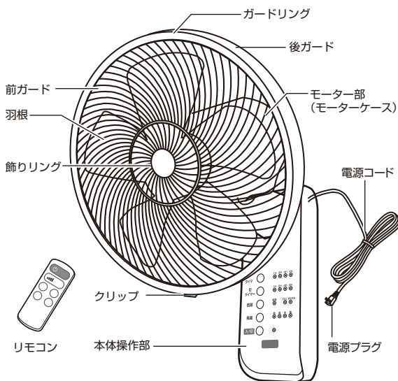
本体
