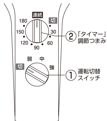
本体操作部
