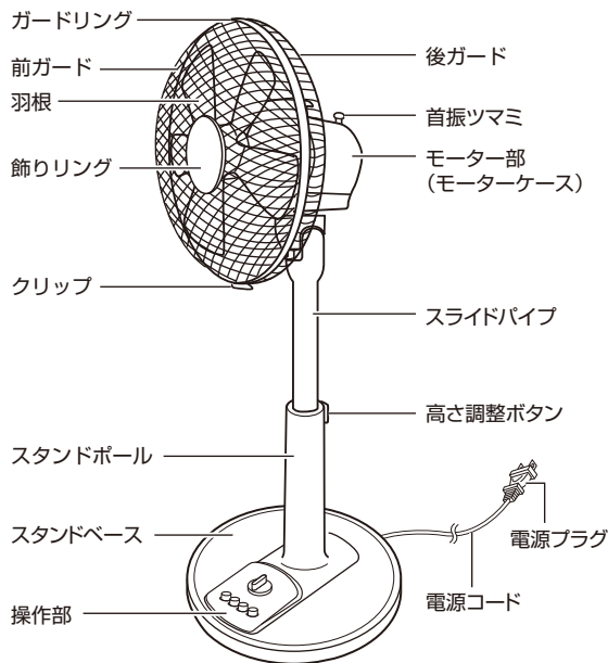
本体
