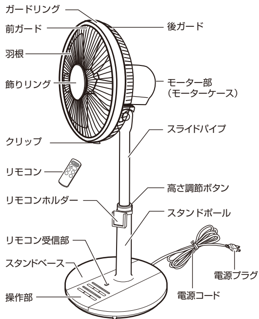
本体操作部
