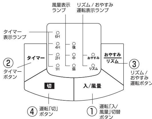
本体操作部
