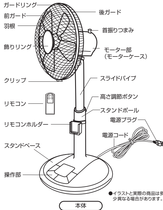
本体
