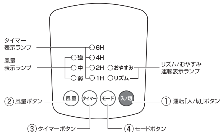
本体:操作部拡大図
