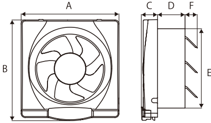
寸法図
